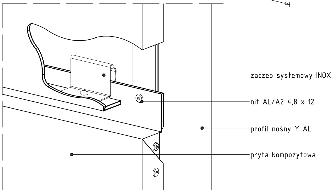
System FORTIS Y - Zaczepowy; widok.
